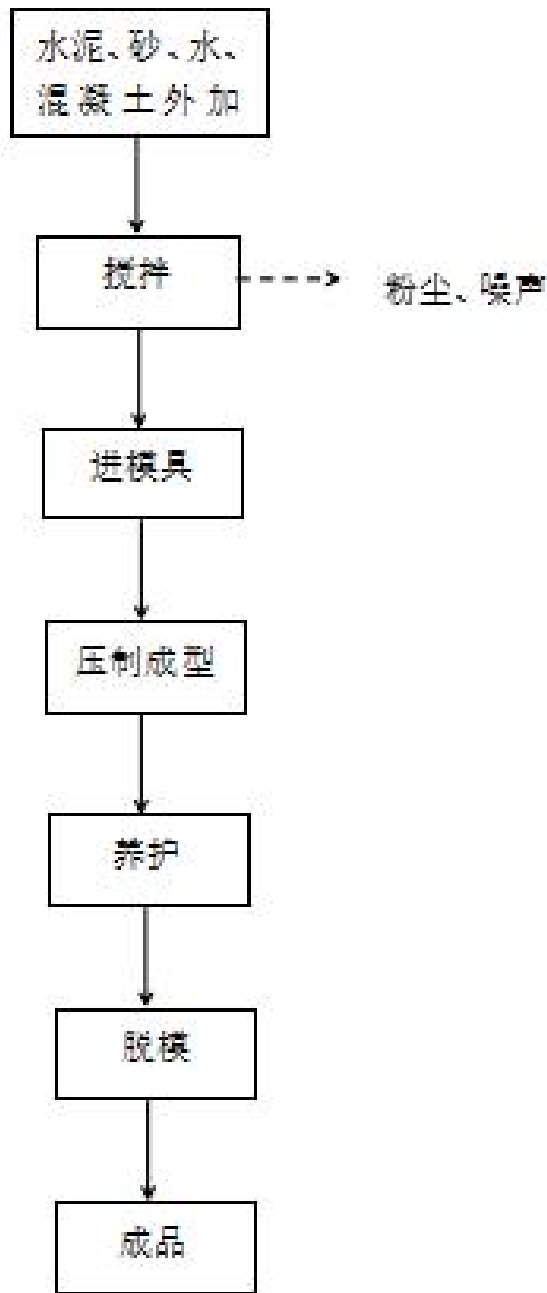
图一 项目生产工艺流程图
