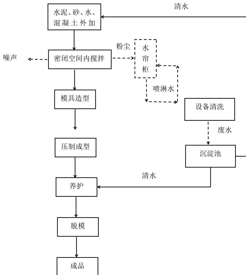
图 1 本项目生产流程及产污节点图
